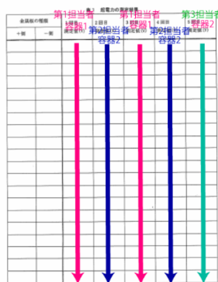
1. 実験1 ボルタ電池と金属のイオン化傾向
